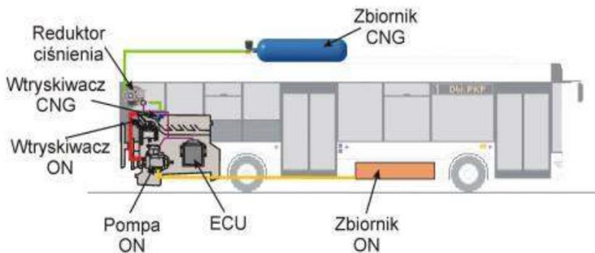
Rysunek 33. Autobus z napędem hybrydowym ON i CNG, źródło: https://cng.lng.pl/wiadomosci/Wspolpraca-z-gazem-wtle,wiadomosc,374.htm
